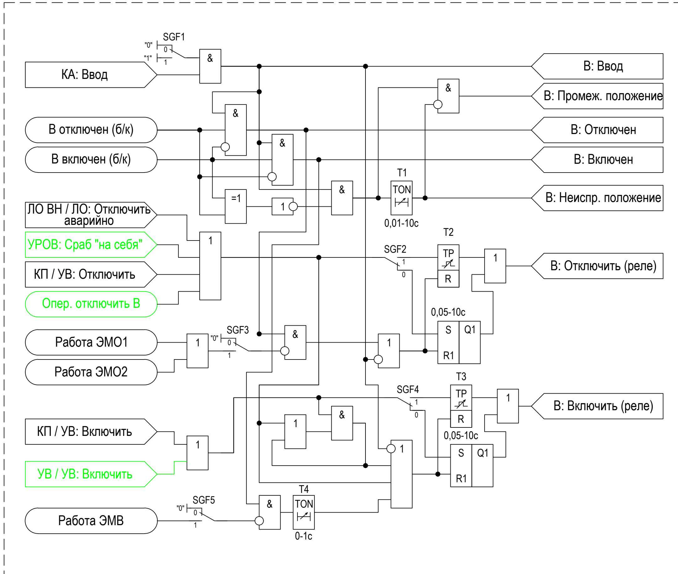
Выключатель (В) (LVCBXCBR) XCBR1
