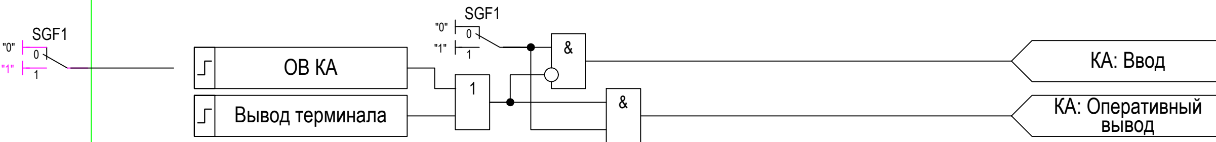
Выключатель (В) (LVCBXCBR) XCBR1
